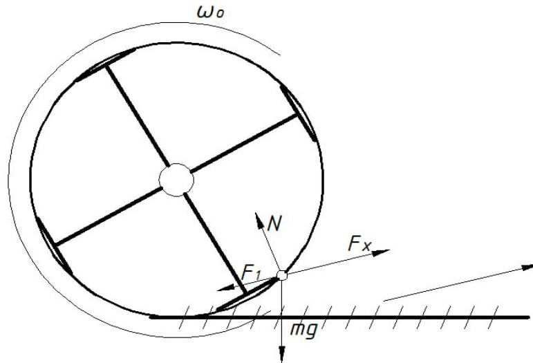
5-rasm. Nazariy tahlillar asosida takomillashtirilgan cho'tkali barabanli titish-tozalash uskunasi
