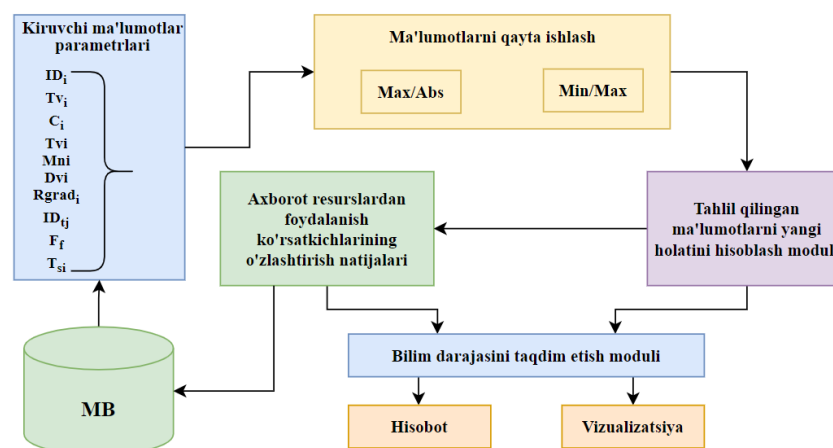
2-rasm. Axborot resurslaridan foydalanish ko'rsatkichlarini baholash sxemasi
